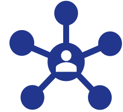
Peer-to-Peer
